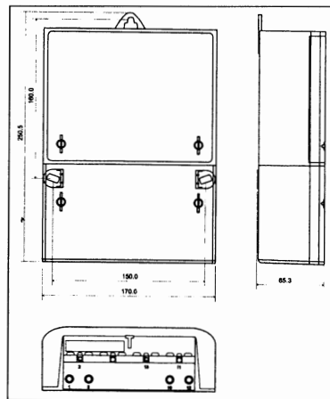
Слика 4 б. Димензије новог кућишта бројила основне ознаке типа ДБ2М
